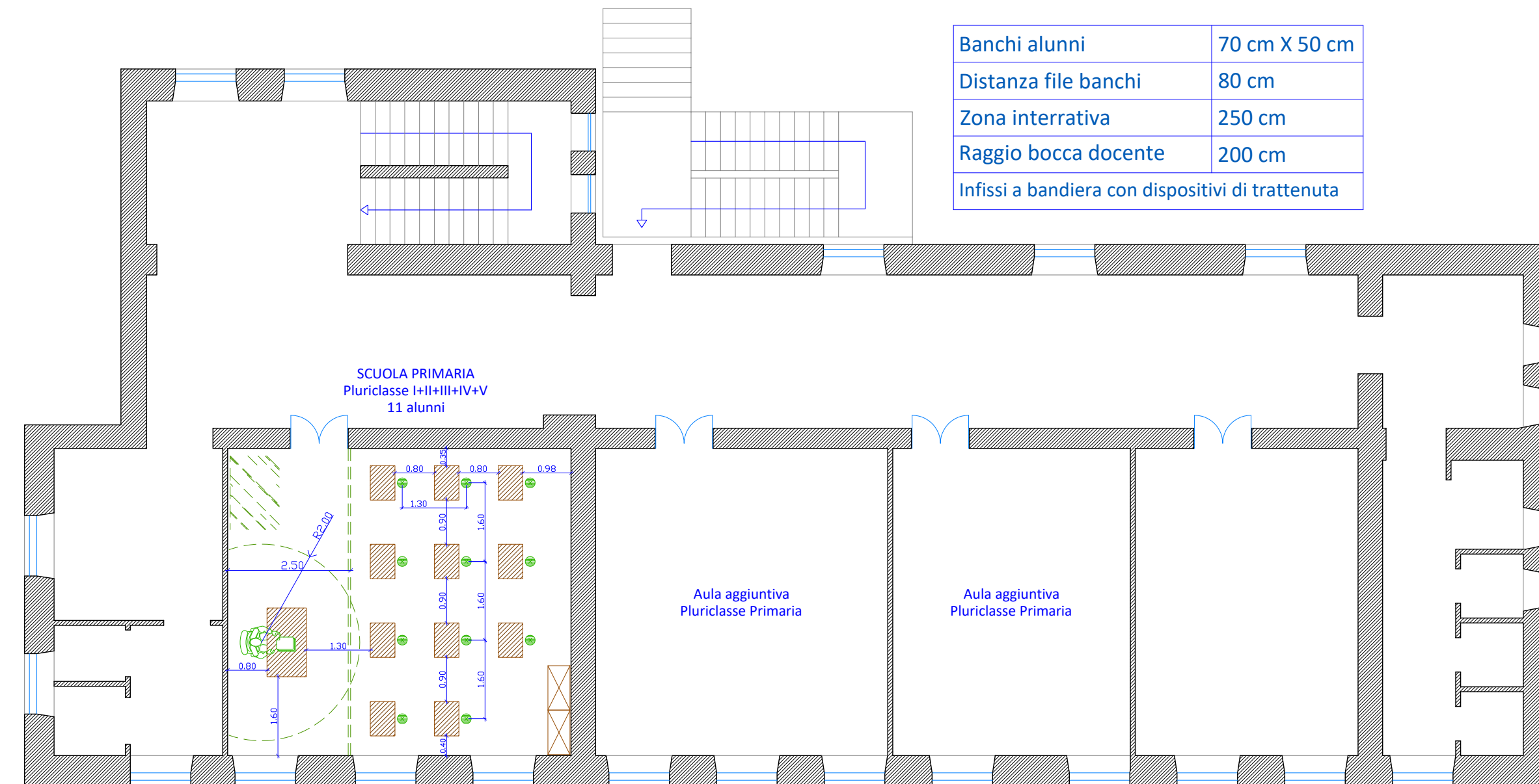
PLESSO CERSOSIMO PIANTA PIANO PRIMO
